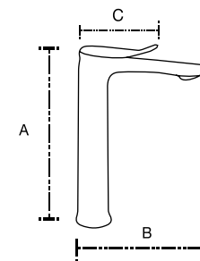
Monomando Lavabo Alto Mod. 75031SB
