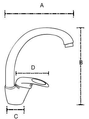
Monomando Fregadero Mod. 6808VCR
