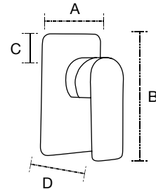
Monomando empotrar para regadera Mod. 73053N
