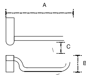
Cepillo de baño cerámico Mod. 70.23031
