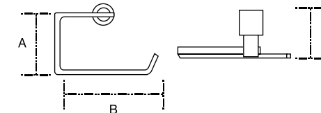
Toallero anilla Mod. 0204
