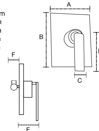
Monomando empotrar Regadera Mod. 65.1302
