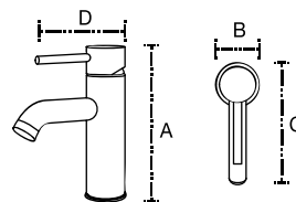
Monomando Fregadero Mod. 37.1043CR
