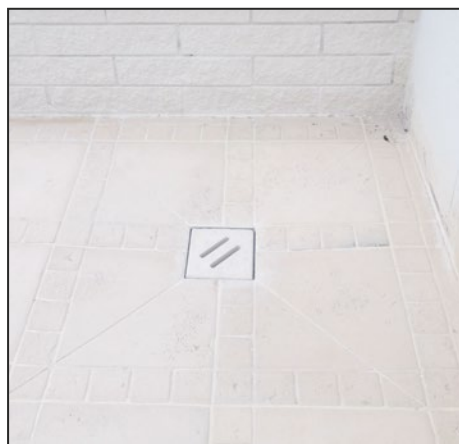
Ángulo drenaje/ducha NERJA solaneta
