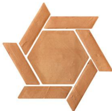
Combinación Firenze Hexágono 19,5 x 22 x 2 cm + Lacería 4,8 x 17 x 2 cm AL-870
