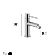
Grifería para bidé cuerpo liso*
