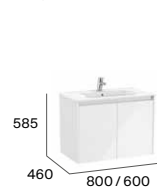
Unik (lavabo y mueble) con puertas
